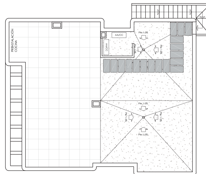
PLANTA CUBIERTA
