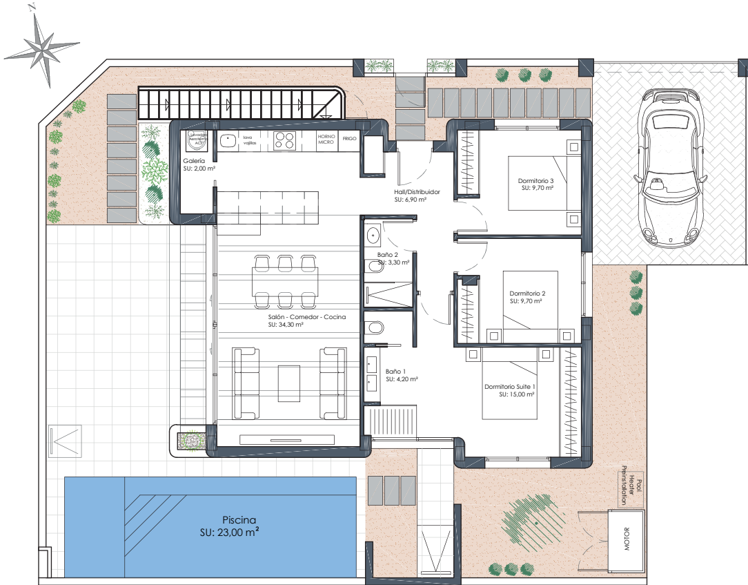
PLANTA BAJA
