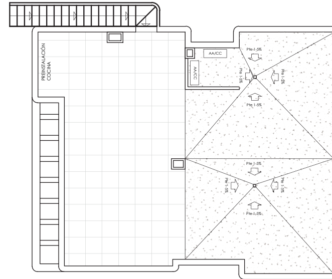
PLANTA CUBIERTA
